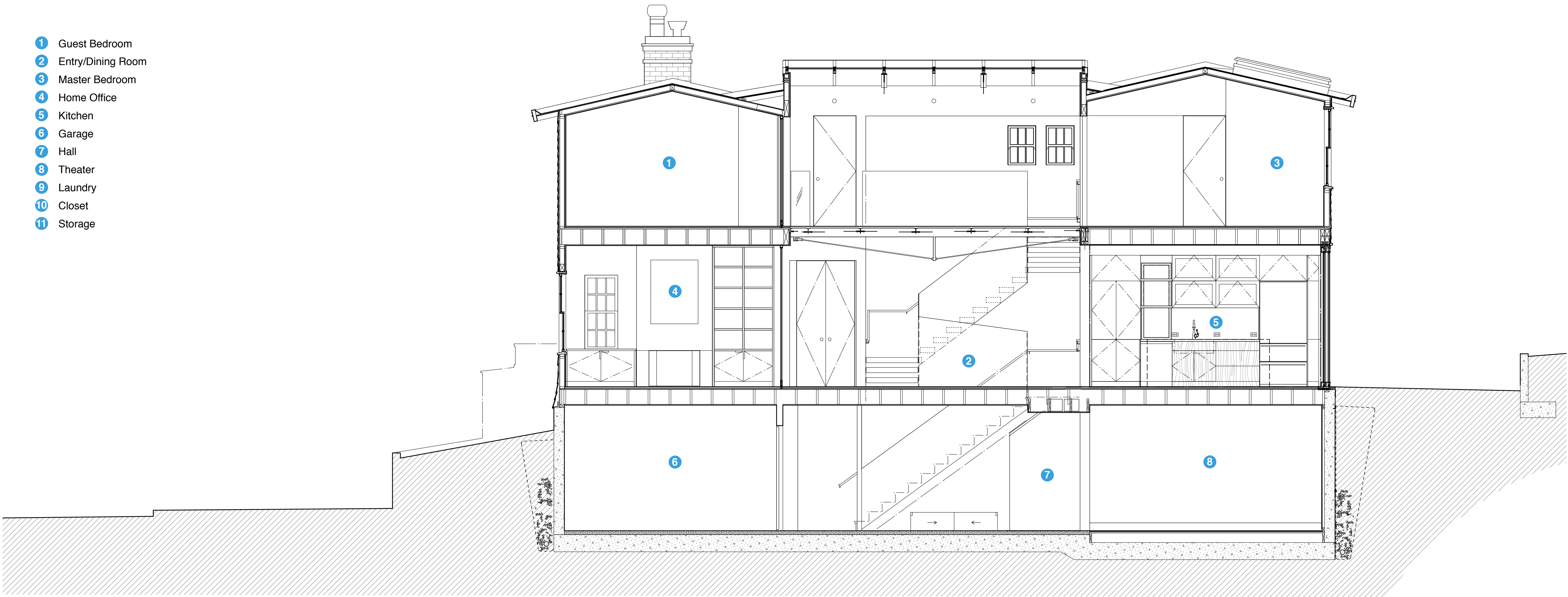
SECTION A-A
